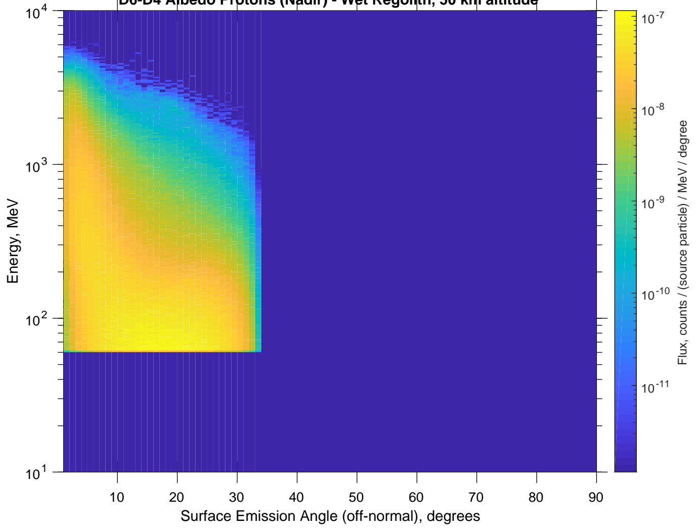
D6-D4 Albedo Protons (Nadir) - Wet Regolith, 50 km altitude
