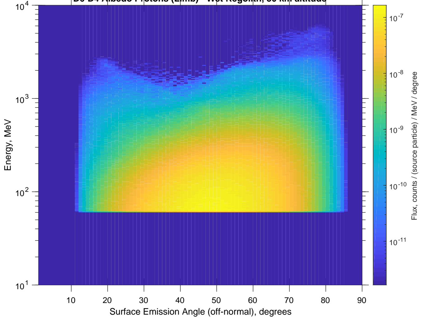
D6-D4 Albedo Protons (Limb) - Wet Regolith, 50 km altitude
